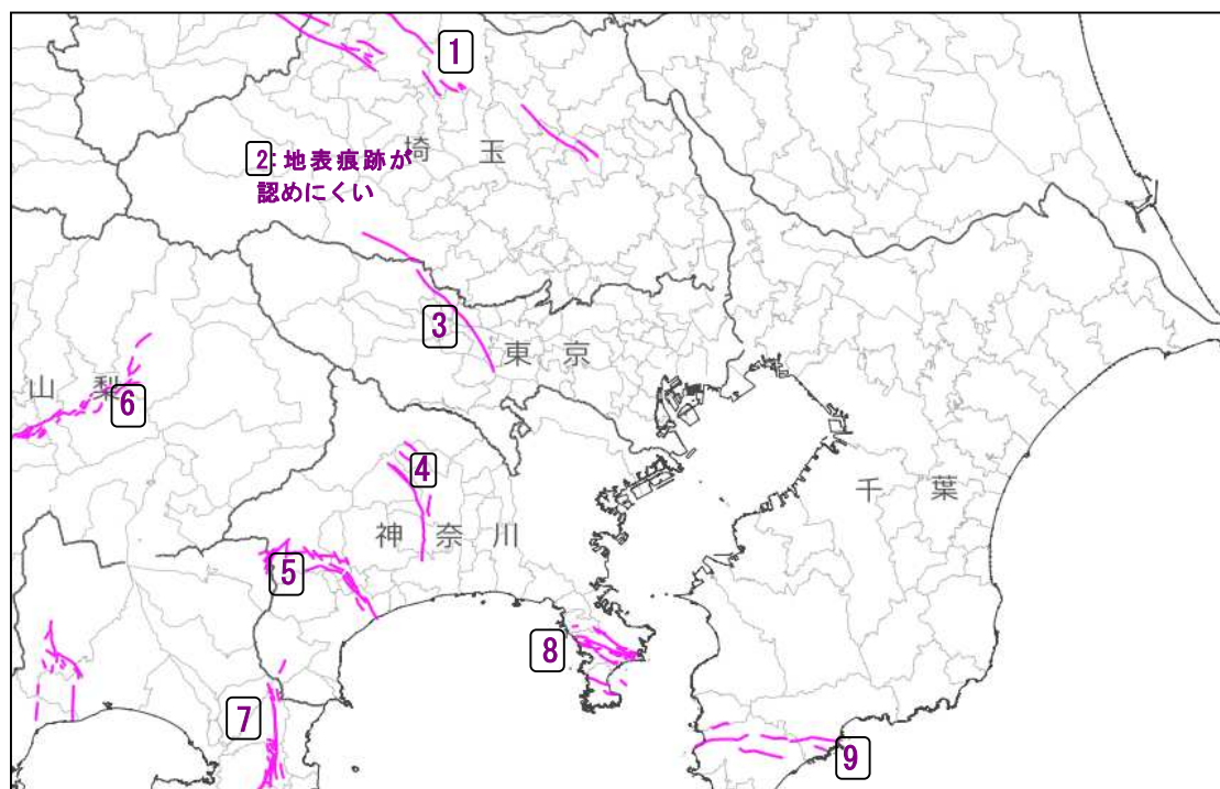
＜南関東付近の主要活断層帯＞
