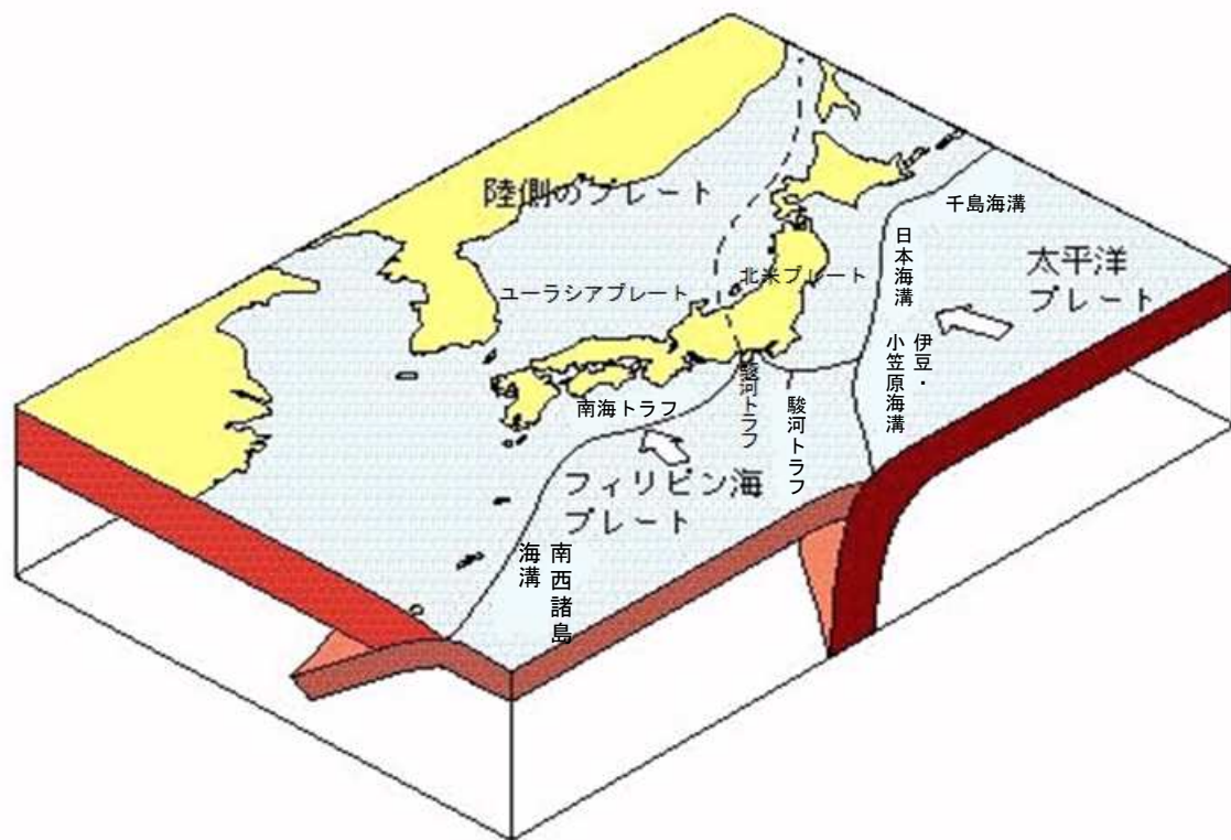
＜日本周辺のプレート分布＞
