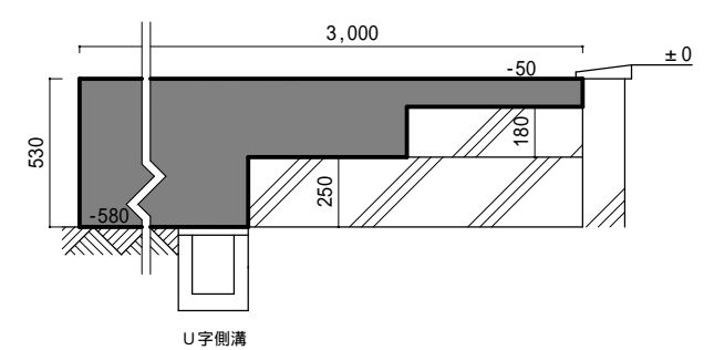
プラットフォーム断面図 1/30
