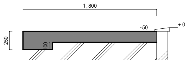
プラットフォーム断面図 1/30
