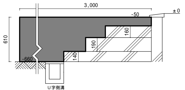
プラットフォーム断面図 1/30
