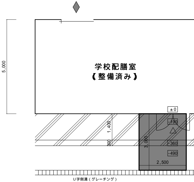
プラットフォーム ( 2,500 × 3,000 × H440 ) 【 指定整備 ( 事業者 ) 】
