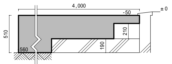
プラットフォーム断面図 1/30
