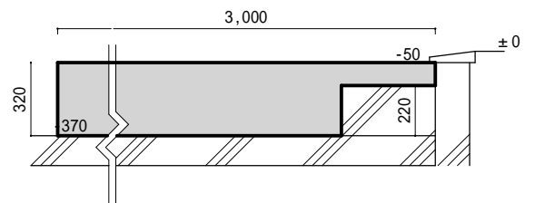
プラットフォーム断面図 1/30
