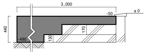
プラットフォーム断面図 1/30
