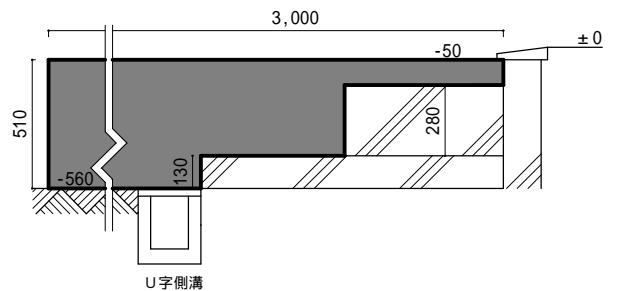
プラットフォーム断面図 1/30
