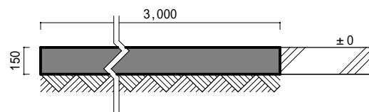
プラットフォーム断面図 1/30
