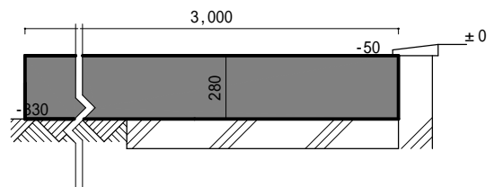
プラットフォーム断面図 1/30
