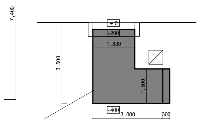
プラットフォーム (3,500×3,000×H400) 【指定整備(事業者)】
