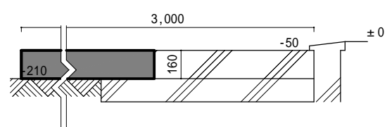
プラットフォーム断面図 1/30
