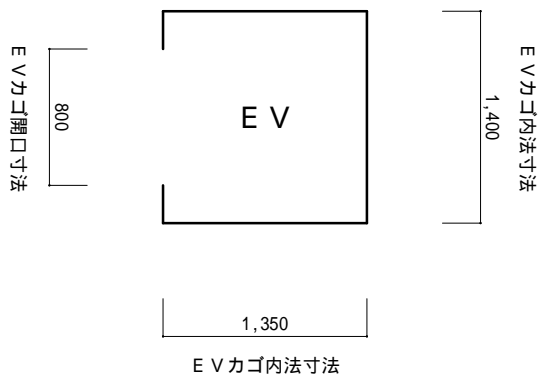
EV平面図 (参考) 1/50
