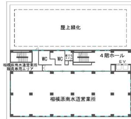
4階平面図 S=1/500
