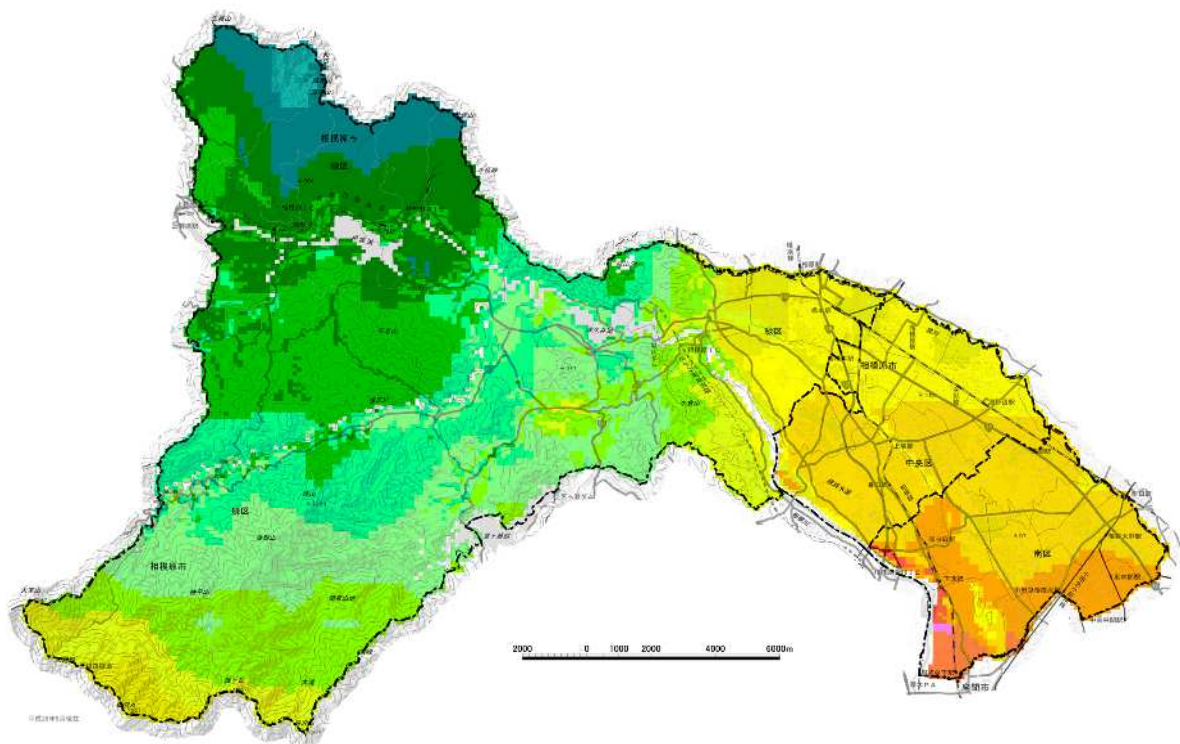
<震度分布図>
