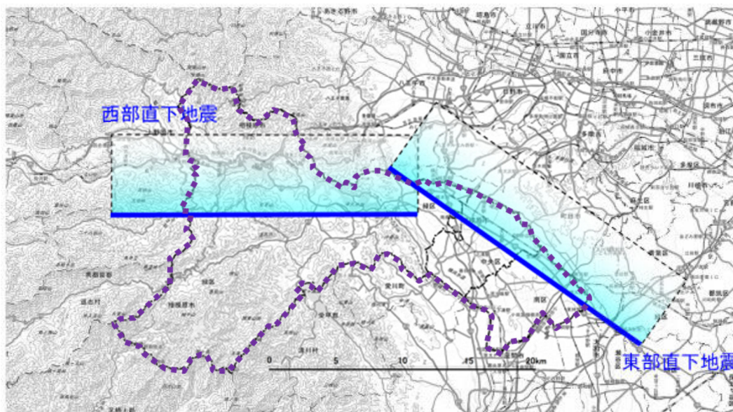
図2-1 想定した震源断層の位置(相模原市東部直下及び西部直下の地震。なお、大正関東タイプの地震の震源域は、相模原市を含む南関東一帯の直下に広がっています。)
