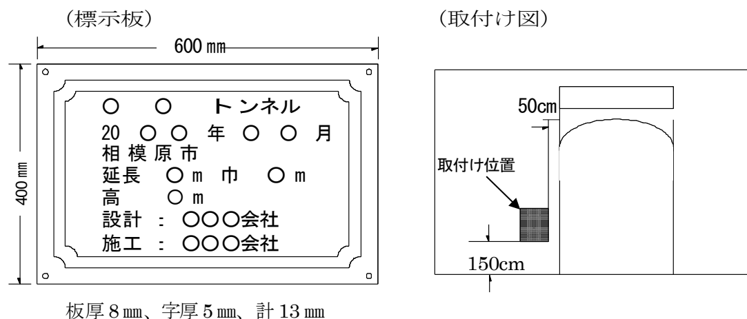
図6-2 設置イメージ図
