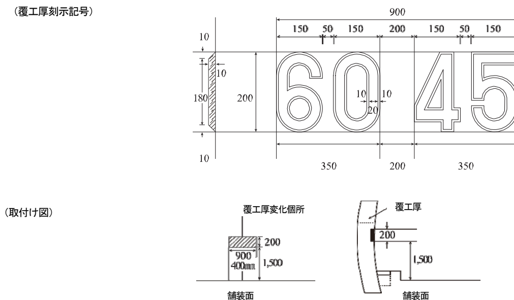
図6－1 覆工厚変化箇所の刻示標準図
